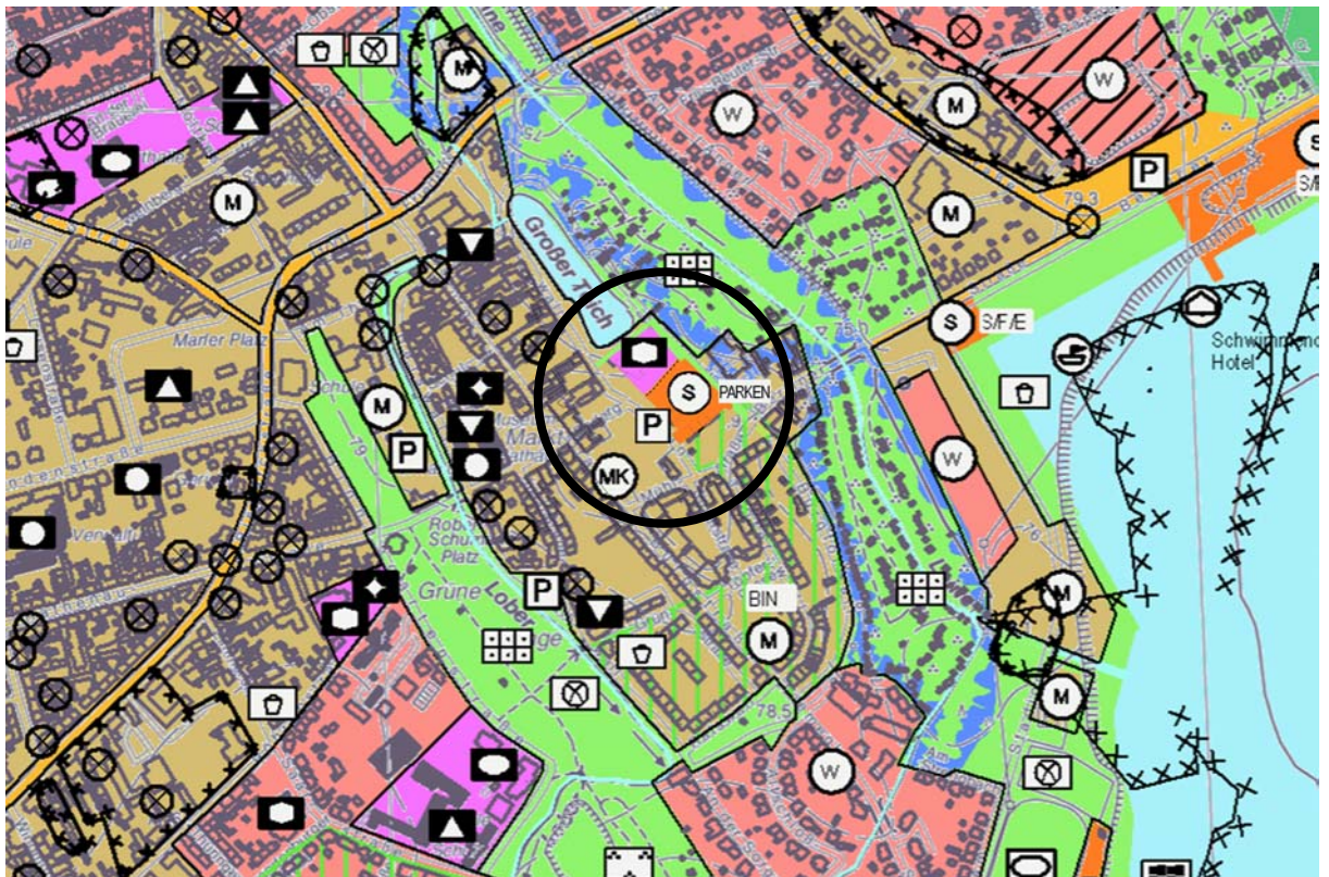
Berichtigung Flächennutzungsplan der Stadt Bitterfeld-Wolfen (Auszug) M 1: 10.000
