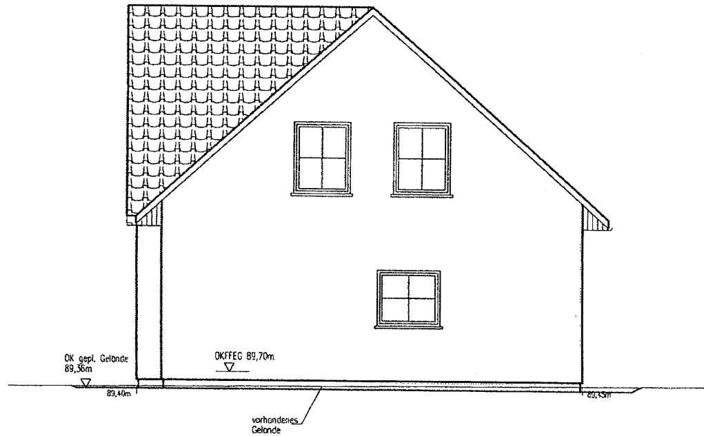
West- Ansicht
