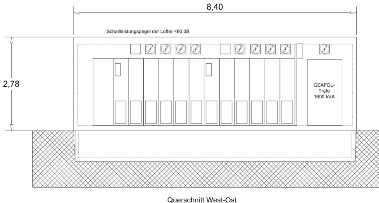
Abb.2: Schema Wechselrichterstation
